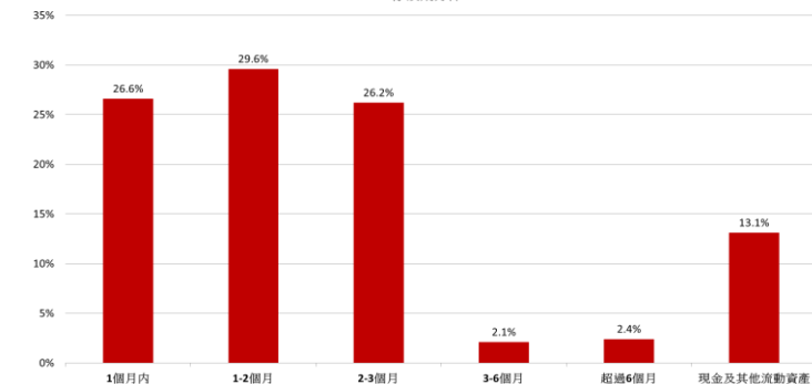
存續期分佈
